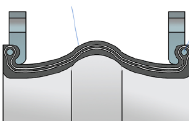
RINFORZO METALLICO METALLIC REINFORCEMENT
